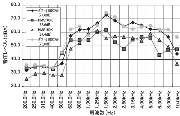
消音特性
