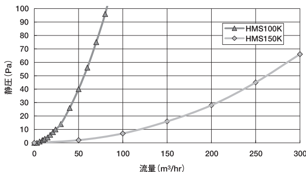
通気性能
